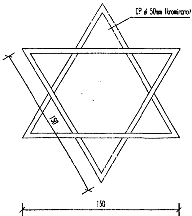
DAVIDOVA ZVIJEZDA-DETALJ
