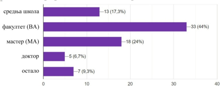
Графикон 4. Школска спрема испитаника
