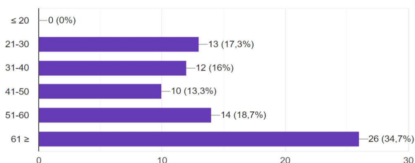
Графикон 2. Старосна структура испитаника
